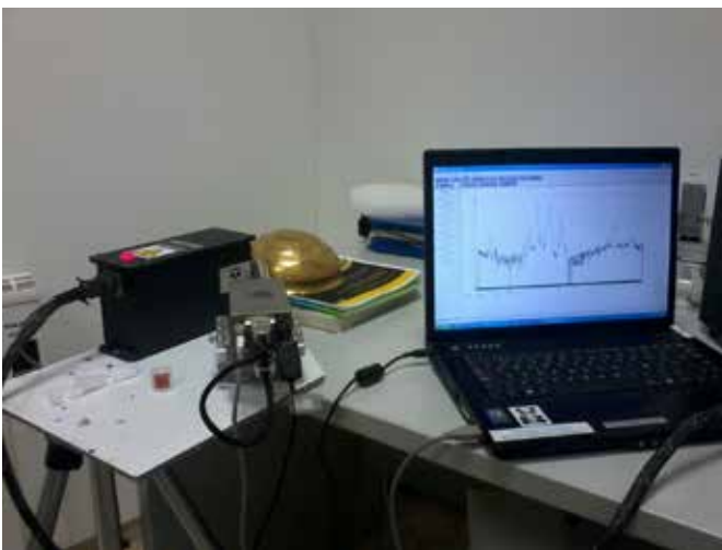
Análisis con tubo de rayos X a un cuenco del Tesoro de Villena.
